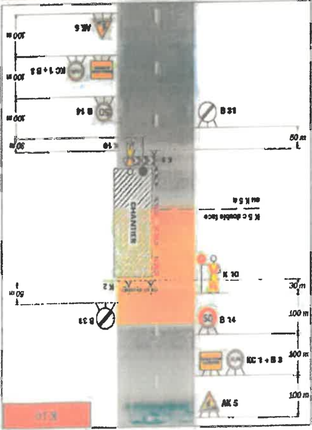
Schémas signalisation temporaire pour alternats de circulation
